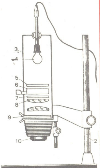
1. გამადიდებლის ეკრანი; 2. შტანგი; 3. გამანათებლის გარსაცმი; 4. ნათურა; 5. თბოფილტრი; 6. შუქფილტრების ჩარჩო; 7. მჭრქალი მინა; 8. კონდენსორი; 9. ნეგატივის ჩარჩო; 10. ობიექტივი.
