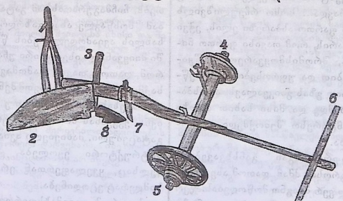
1. მხარი 2. ფრთა 3. ხმალა 4. ველის ვოვორა 5. კვალის ვოვორა 6. უღელი 7. საკეთული 8. სახნისი
