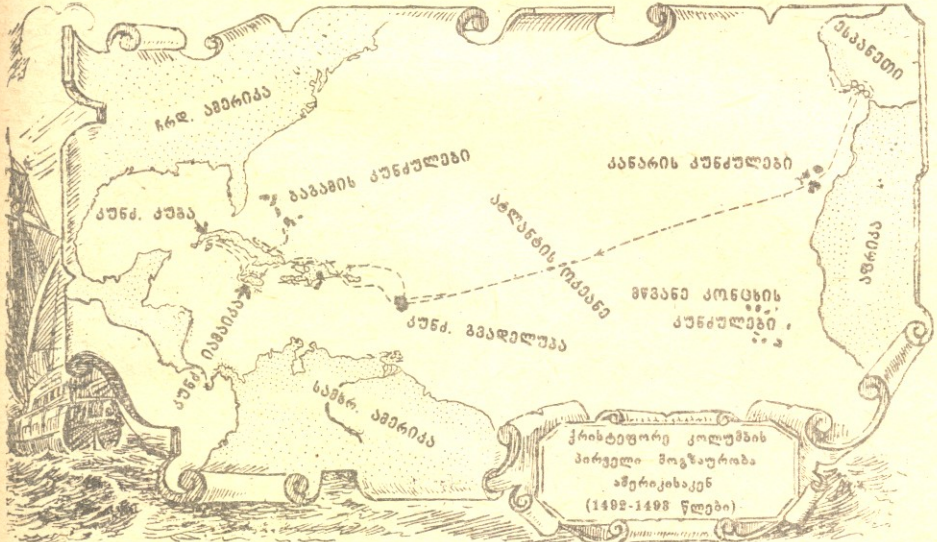
ქრისტოფოროს კოლუმბის პირველი მოგზაურობა აფრიკისაკენ (1492-1498 წლები)
