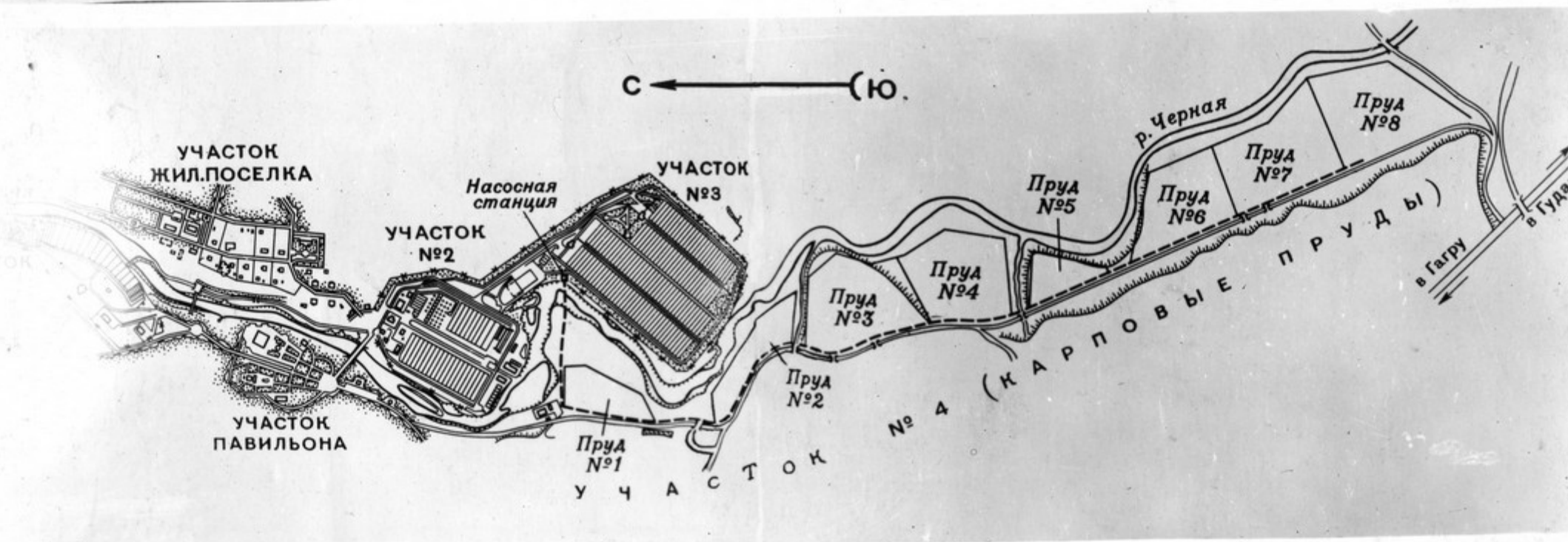
Генеральный план хозяйства.
