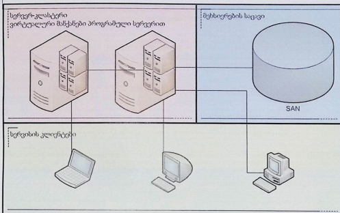
ნახ. 1-მე წარმოდგენილია აღწერილ ტექნოლოგიათა კომბინირებით აგებული სერვერული სისტემის მარტივი ნიმუში.
