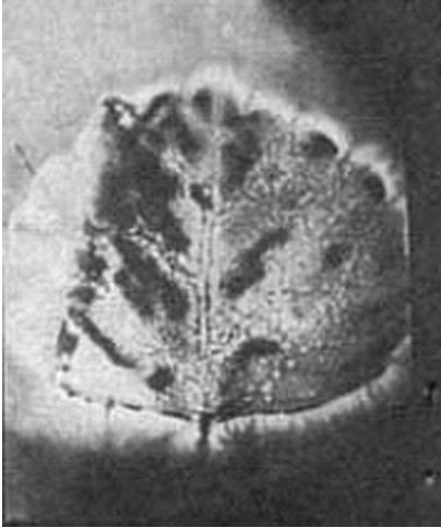
პირლიანის ფოტოეფექტი
