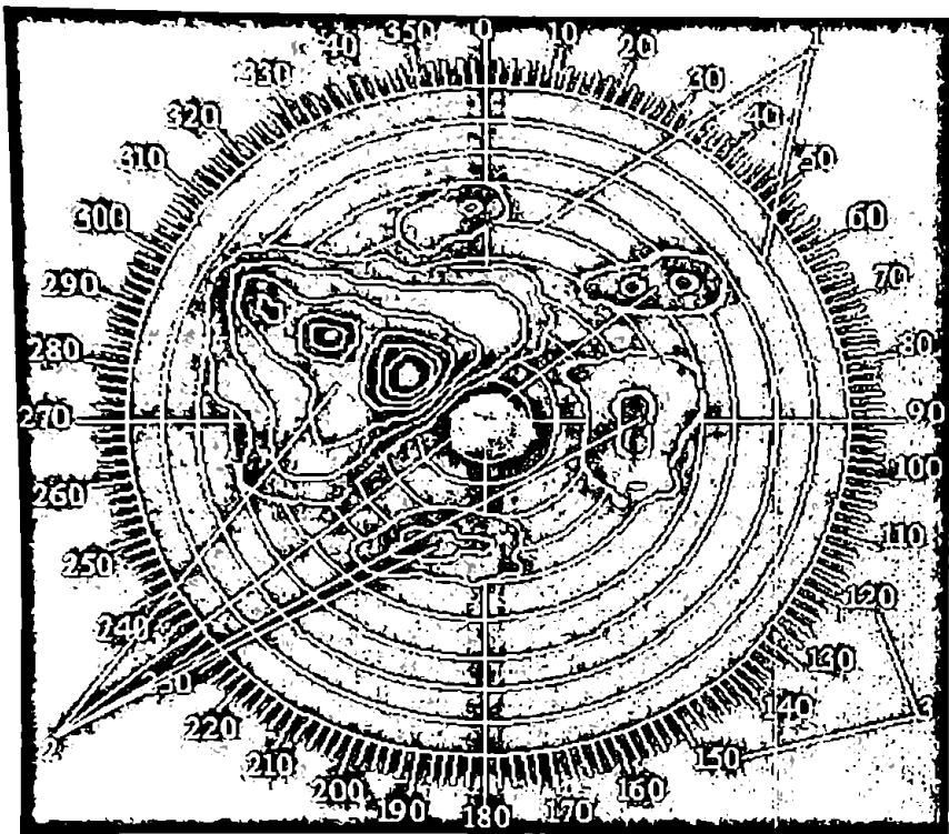
ნახ. 2. სეტყვის ღრუბლის რადიოქოს დისკრეტული გამოსახულების ფოტო. 1-მანძილის კვლები; 2-ღრუბლის რადიოქო; 3-აზიმუტური შკალა. მანძილის კვლები შეესაბამება 5კმ-ს.
