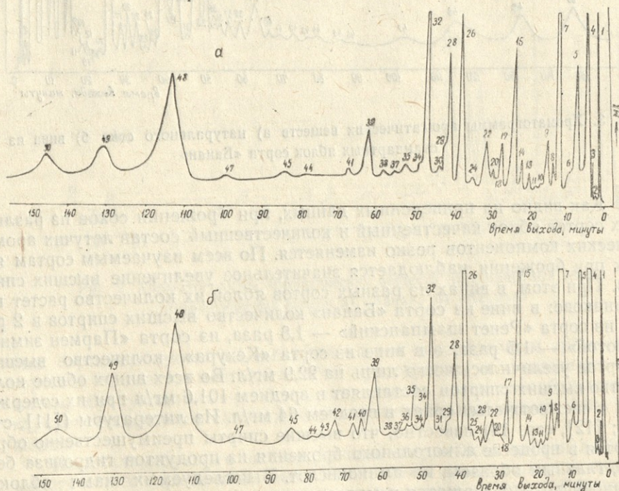
Рис. 5. Хроматограммы ароматических веществ а) натурального сока, б) вина из нестандартных яблок сорта «Пармен зимний золотой».
