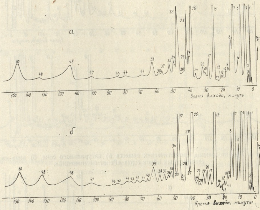
Рис. 3. Хроматограммы ароматических веществ а) натурального сока б) вина из нестандартных яблок сорта «Банан»
