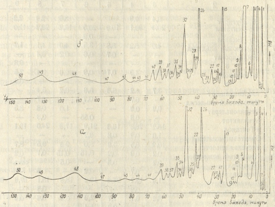
Рис. 6. Хроматограммы ароматических веществ а) натурального сока, б) вина из нестандартных яблок сорта «Кехура».
