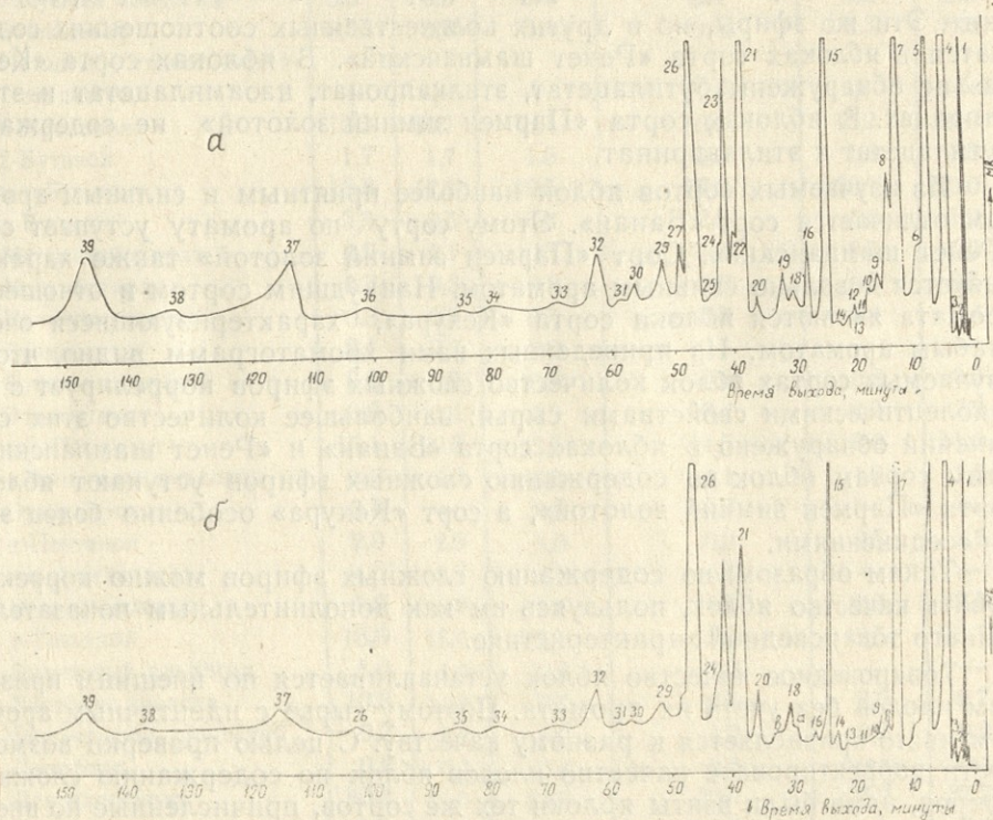
Рис. 2. Хроматограммы ароматических веществ нестандартных яблок помолологических сортов а) «Банан» б) «Кехура»
