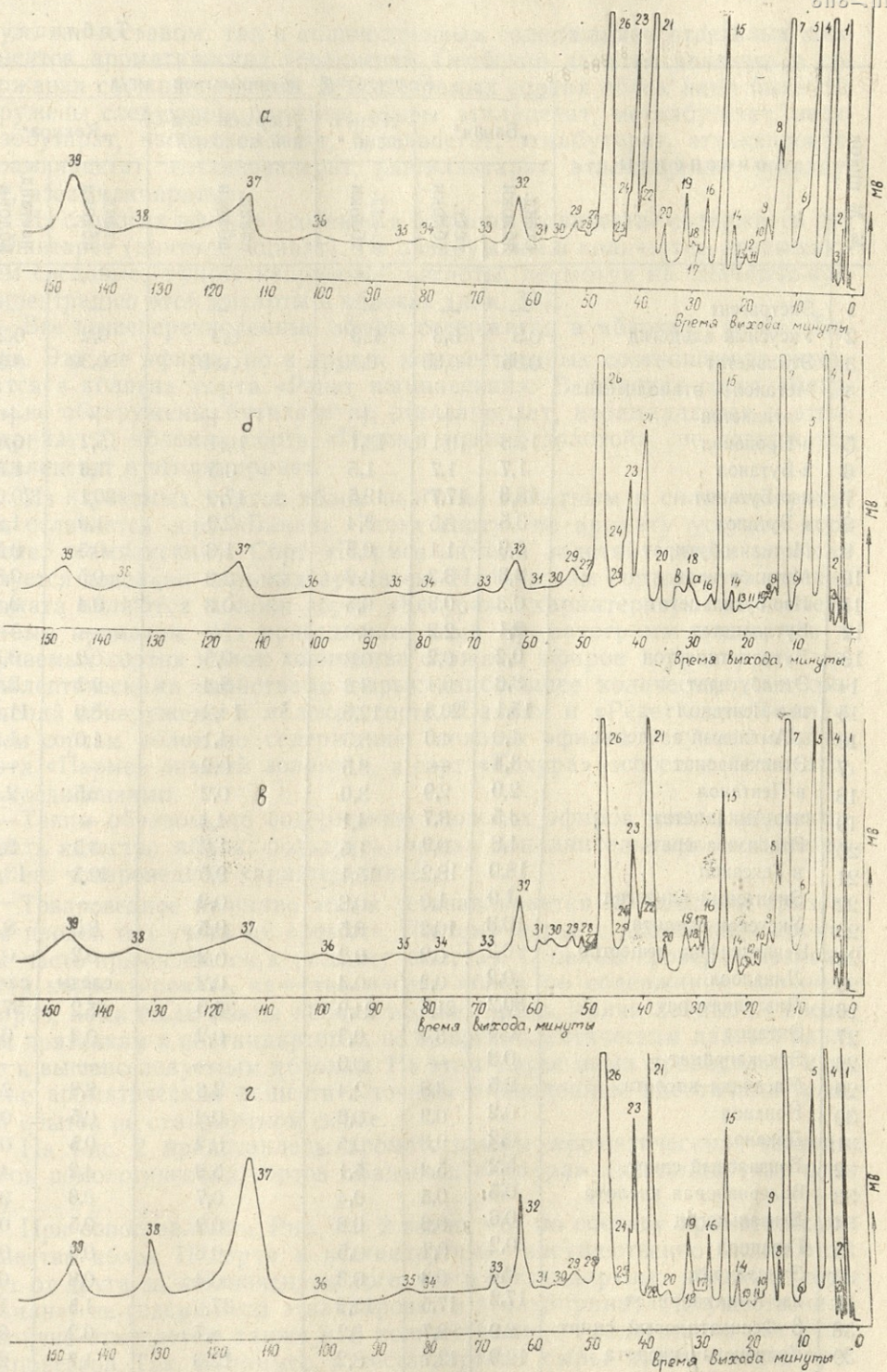
Рис. 1. Хроматограммы ароматических веществ яблок различных помологических сортов а) «Банан» б) «Кехура» в) «Ренет шампанский» г) «Пармен зимний золотой».
