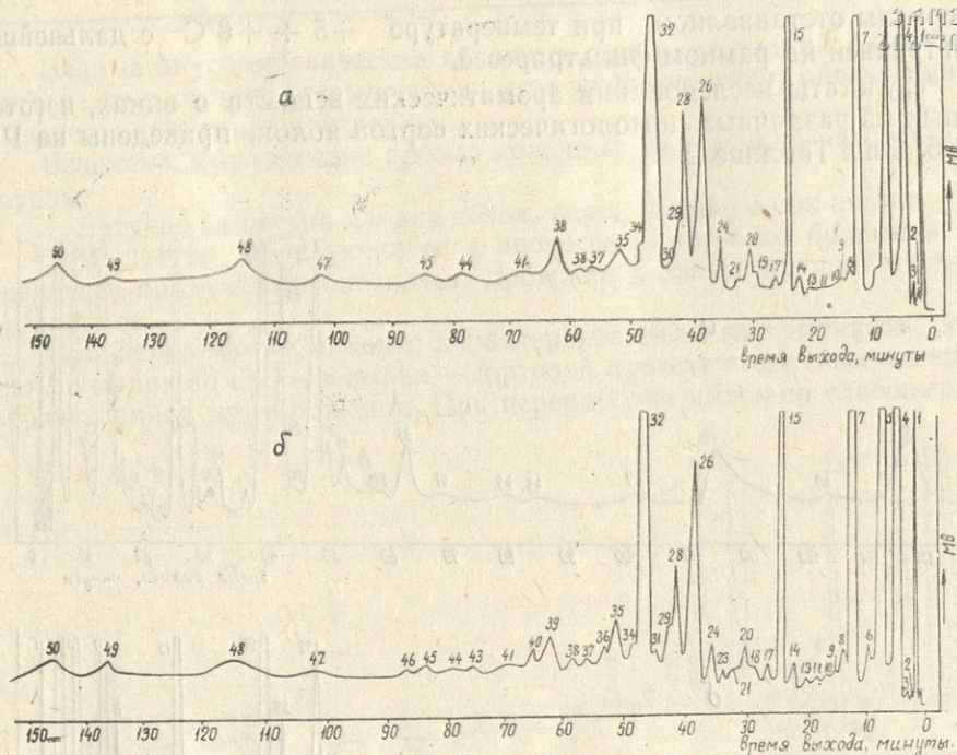
Рис. 4. Хроматограммы ароматических веществ а) натурального сока, б) вина из нестандартных яблок сорта «Ренет шампанский».
