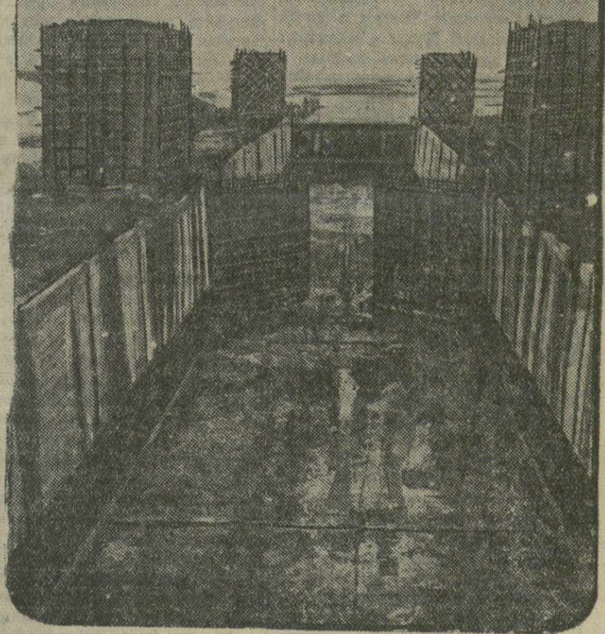
Канал Москва — Волга. На снимке: Карамышевский шлюз. (Фото Ф. Кислова—Союзфото).
