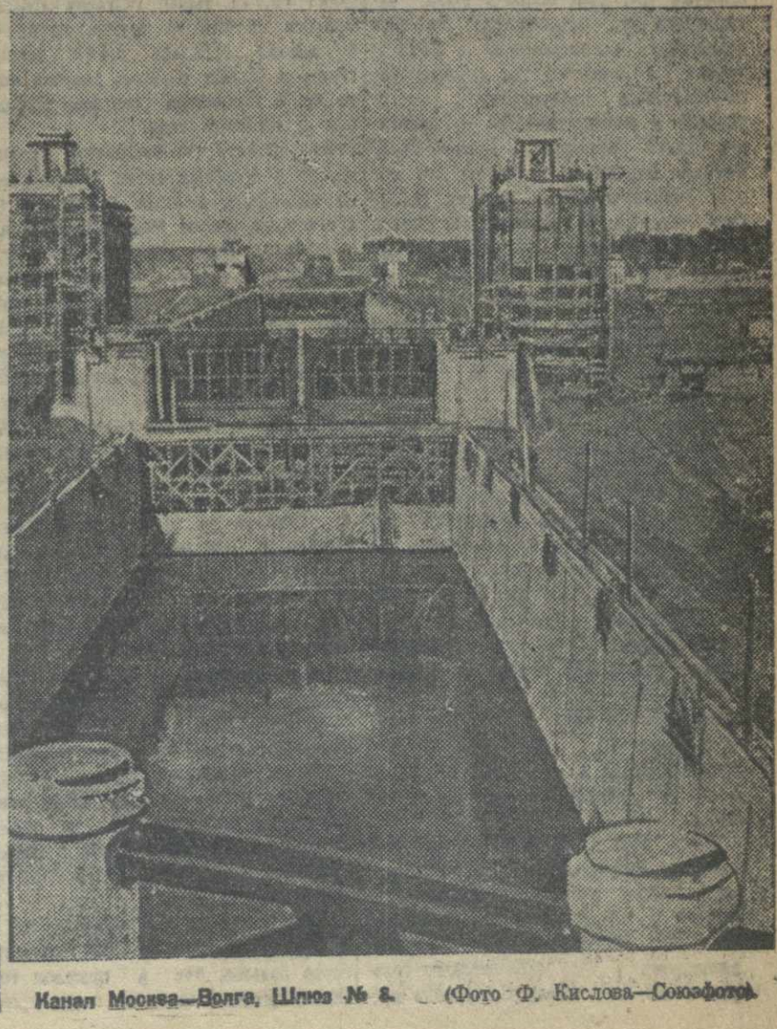
Канал Москва—Волга, Шлюз № 8. (Фото Ф. Кислова—Союзфото).
