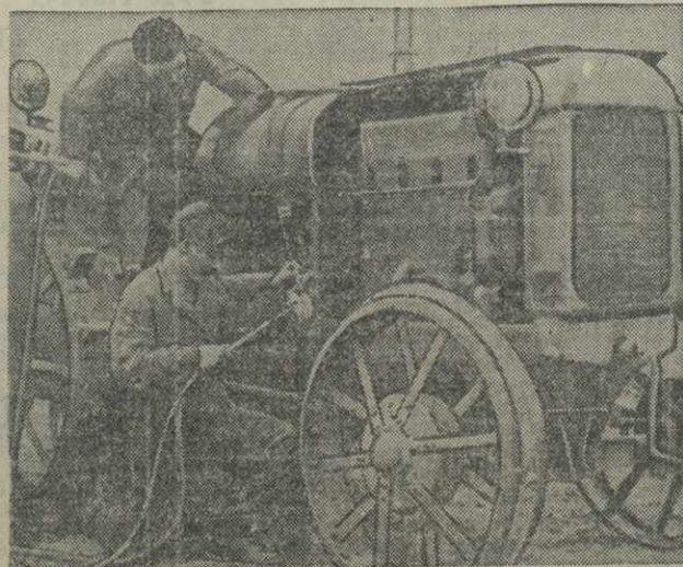
Автогенная сварка корпуса трактора «СТЗ» на Каспской МТС. (Фото В. Полякова).
