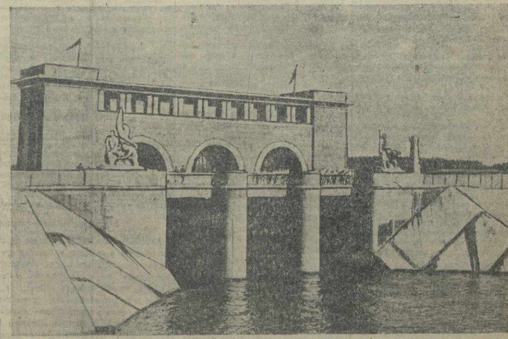
На участках канала Москва — Волга заканчиваются приготовления к паводку. Шлюзы и прочие сооружения осмотрены и подготовлены к новой навигации, открытие которой ожидается в конце апреля. На снимке: водосбор Пестовской плотины. (Фото Р. Дюамента — Совфото).
