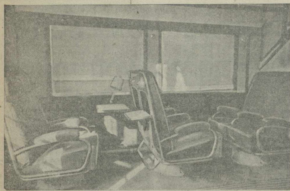
Малининский вагоностроительный завод выпустил образец нового цельнометаллического двадцатипятиметрового мягкого вагона областного сообщения. На снимке: часть вновь выпущенного вагона, установленного в Доме техники НКПС. Фото А. Гусева. Фотокино ТАСС.
