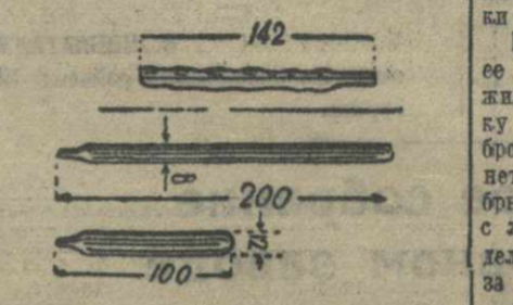
Рисунки № 2. Специальная ампула (верхняя) и ампула (нижняя) для воспламенения смесей № 1 и № 3 (размеры в мм.).
