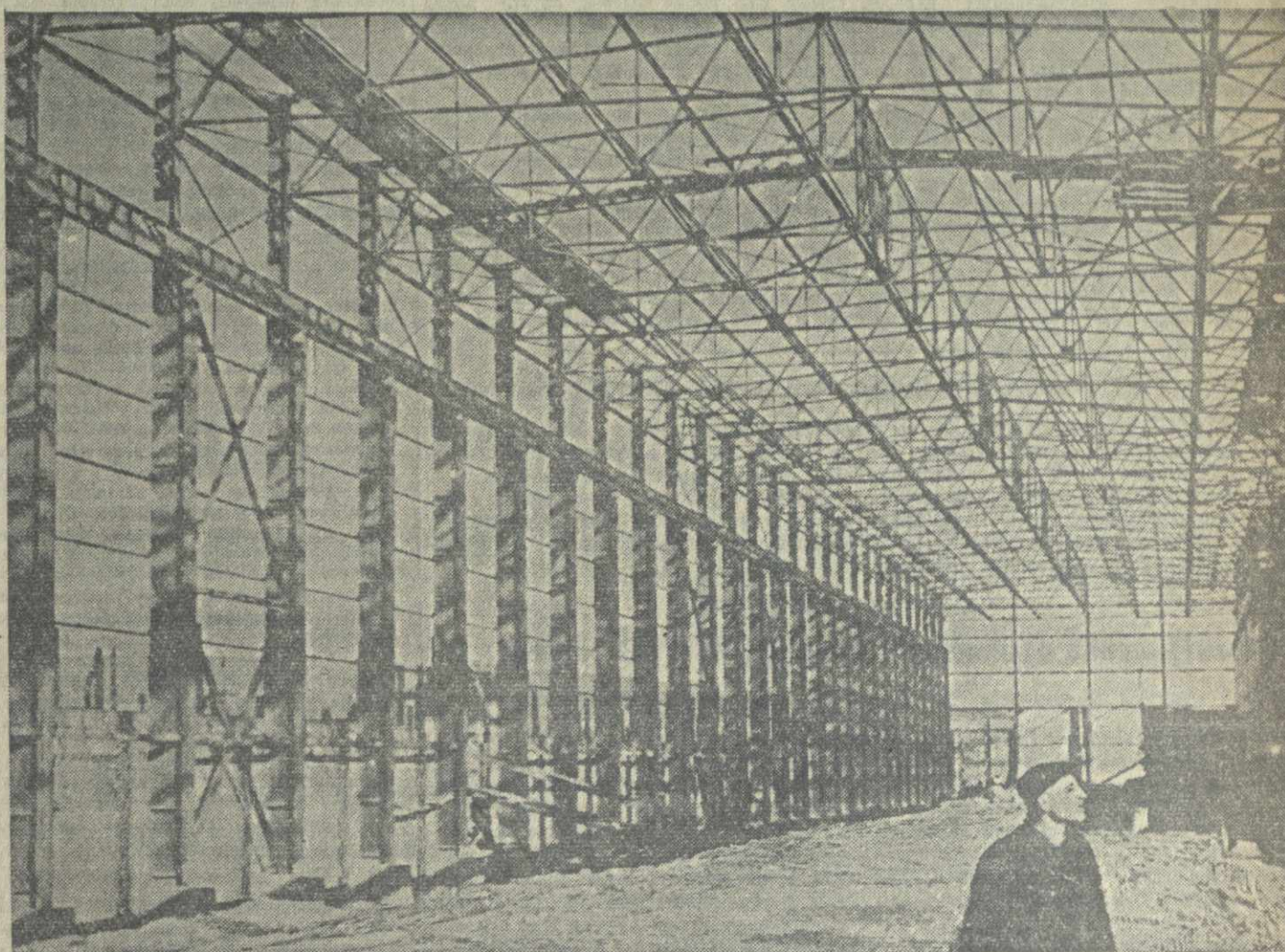
На строительстве Кутанского автозавода. Один из пролетов строящегося блока литейных цехов завода.
