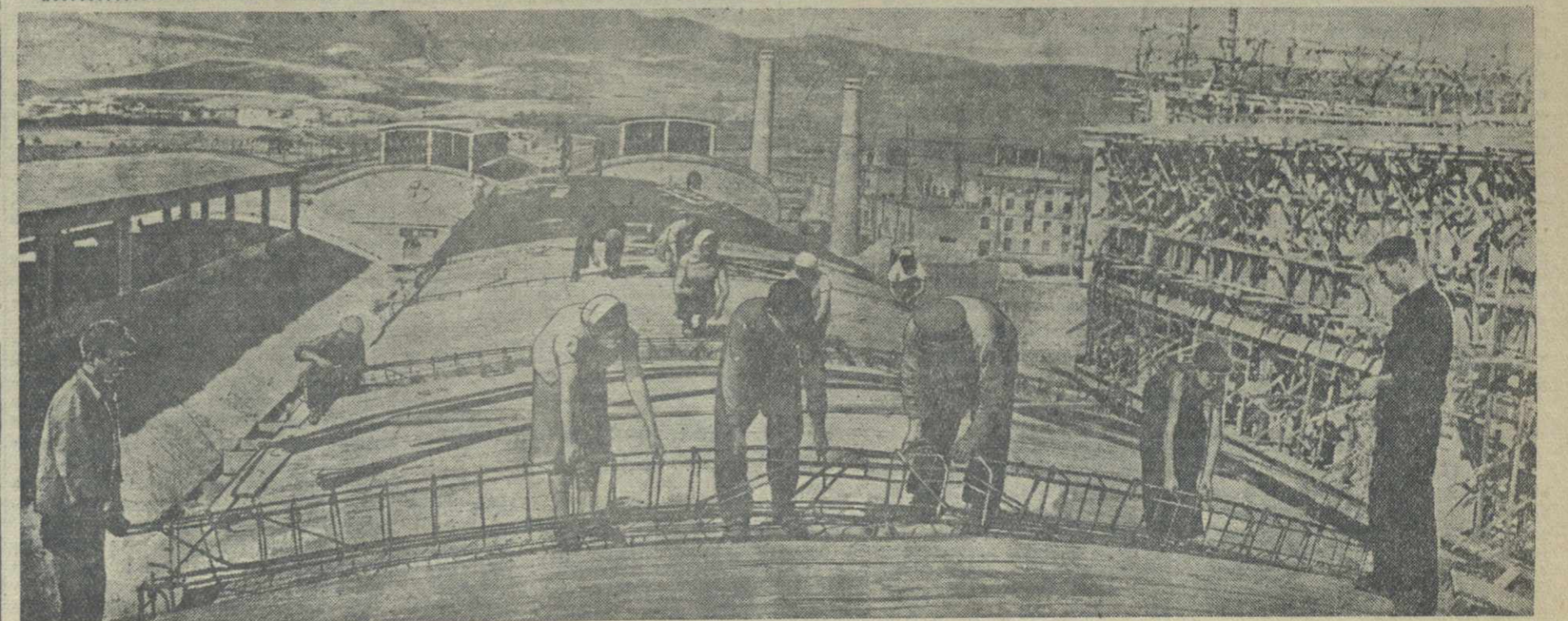
На строительстве электровозоремонтного завода в Авчала. Опалубка крыши корпуса локомотивного депо. Фото В. Тархова.
