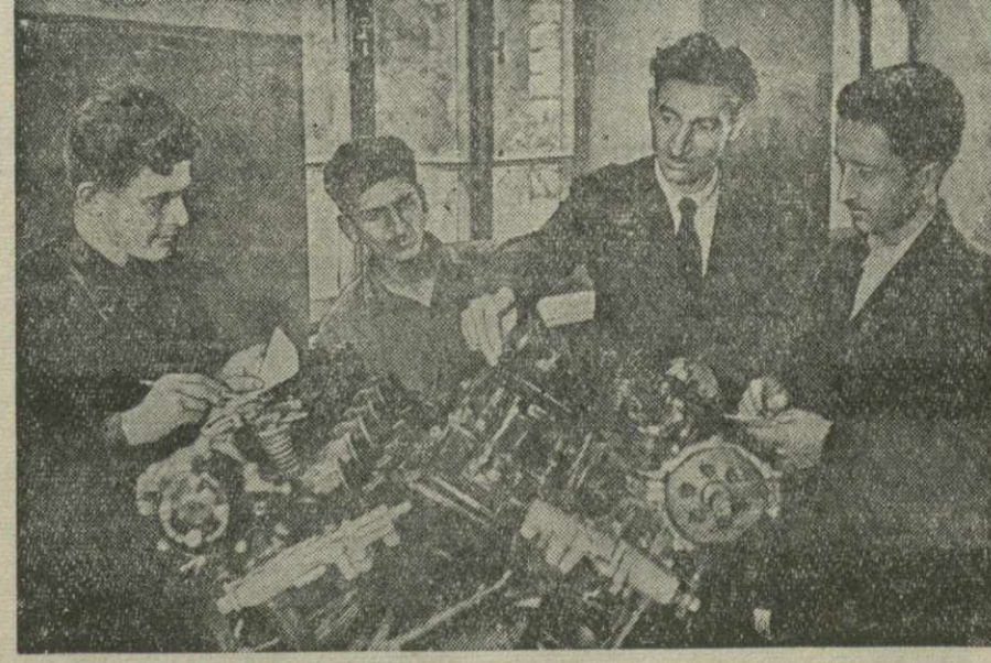
На практических занятиях в Тбилиском авиационном техникуме. Преподаватель инженер С. Давитдзе объясняет студентам взаимодействие частей авиационного мотора. Фото М. Каприкашвили.
