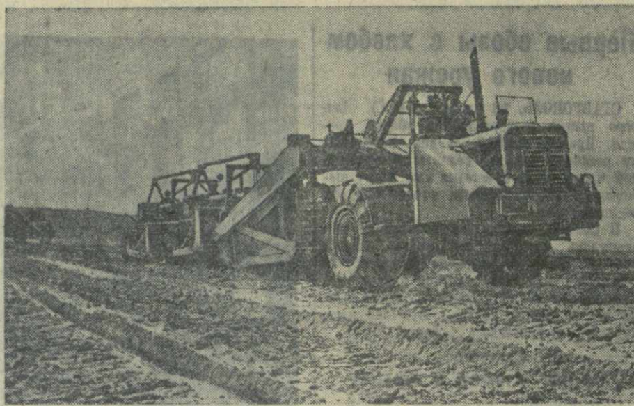
Одна из сверхмощных машин, применяемых для земляных работ в Самгори. Фото В. Тархова.
