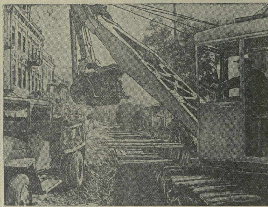
Работы по сооружению ливнеспуска ведутся сейчас на Советской улице. Строители проложили траншею, по которой ливневые потоки пойдут в Куру. На рыхле траншеи работает экскаватор. Вдоль улицы, по которой проходит трасса ливнеспуска, строятся колодцы для приема дождевой воды. В Суидженском озере, на улицах Монтана, Мазунной, Ардовской и 9-го февраля будут построены приемные сооружения, откуда ливневые воды, заливавшие ранее улицы, будут стекать в траншеи. До головных сооружений осталось 400 метров. Строители рассчитывают пройти их к концу года. На снимке: экскаватор на рыхле траншеи для ливнеспуска по Советской улице. Фото В. Гархова.
