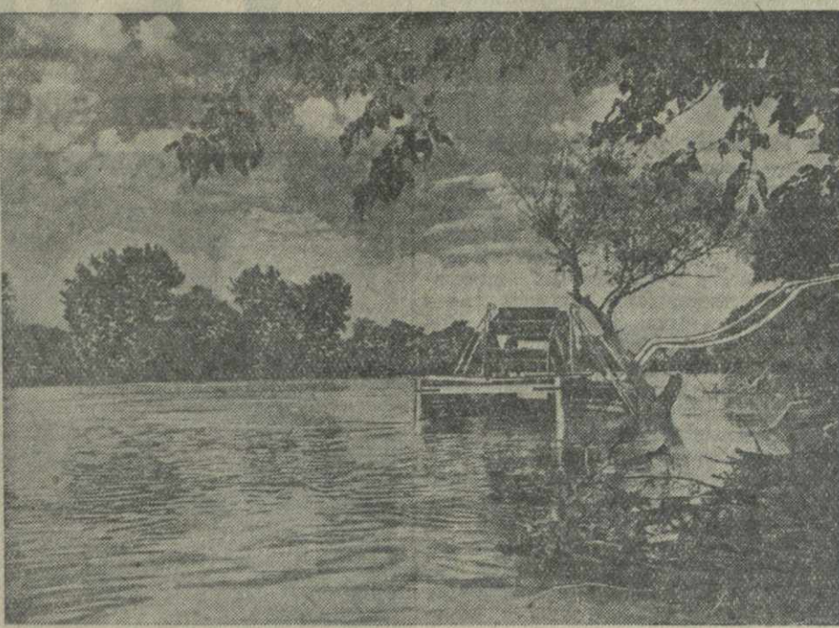
Двухнасосная пловучая станция на реке Алазани, построенная колхозом имени Кирова ссл. Архиласло Цителцакарского района для орошения огородов. Фото П. Луценко.
