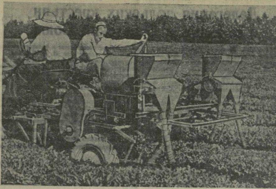
В Лайтурском чайном совхозе имени Кирова проведены испытания чаеформовой самоходной универсальной машины конструкции Всесоюзного института опытного сельскохозяйственного машиностроения. Новая машина выполняет четыре операции: выносит туковые удобрения, рыхлит междурядья, производит подрезку чайных кустов и собирает в бункера чайный лист. На снимке: чаеформовочная машина на плантациях совхоза. Фото В. Бабаяна. Фотохроника ТАСС.
