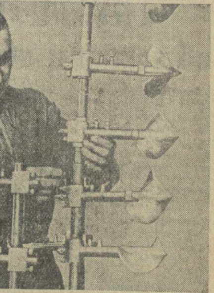
Тбилисский завод «Гидрометр» выполняет заказы великих строек коммунизма. На снимке: слесарь-сборщик Ш. Хуцишвили за сборкой речных вертушек, измеряющих скорость движения воды.
