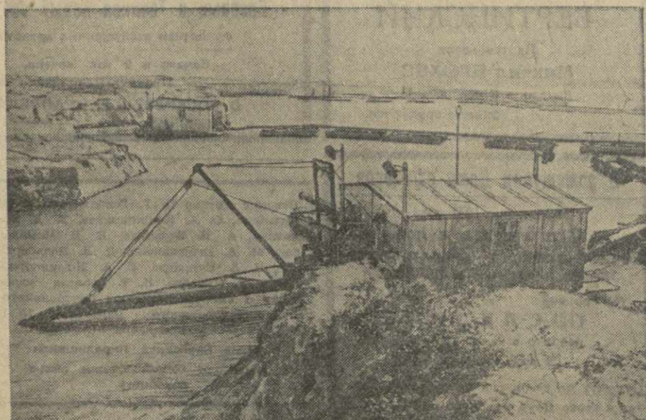
На строительстве Волго-Донского судоходного канала. В районе станции Цимлянской, где будет построено огромное водохранилище, широко развернулись земляные работы по намыву плотины и дамб.
