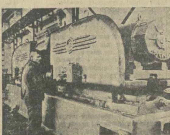
Тбилистский станкостроительный завод им. Кирова впервые в Союзе освоил производство 15-тонного муфто-рас-точного станка. Он предназначен для нефтяной промышленности. На снимке: новый станок образца 1950 года. Фото В. Черкасова.
