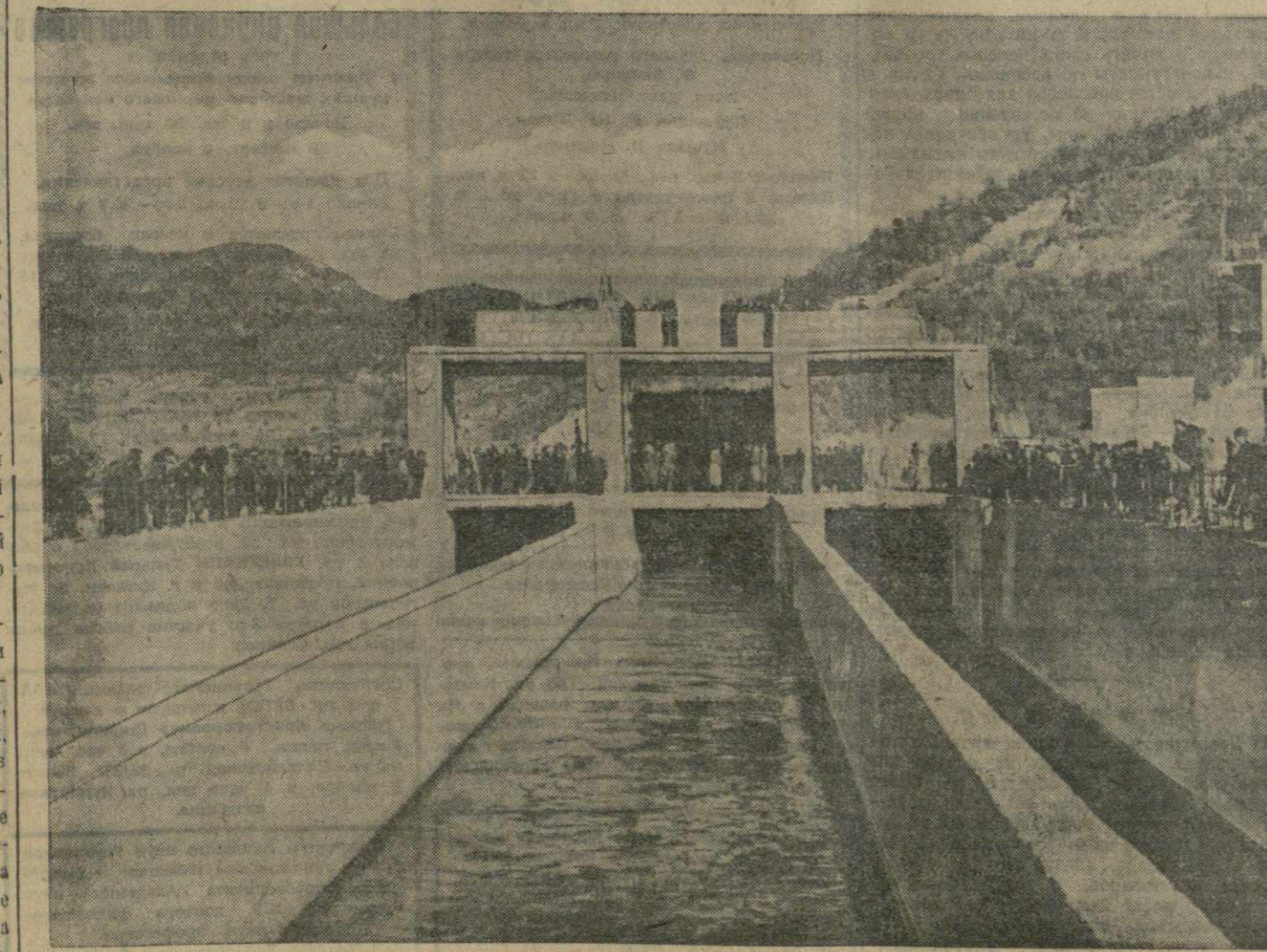
Самгори. Головное сооружение Верхне-Магистрального канала. Щит водоприемника поднят, и воды р. Иори устремились по каналу. Снимок сделан 3 ноября 1951 года.
