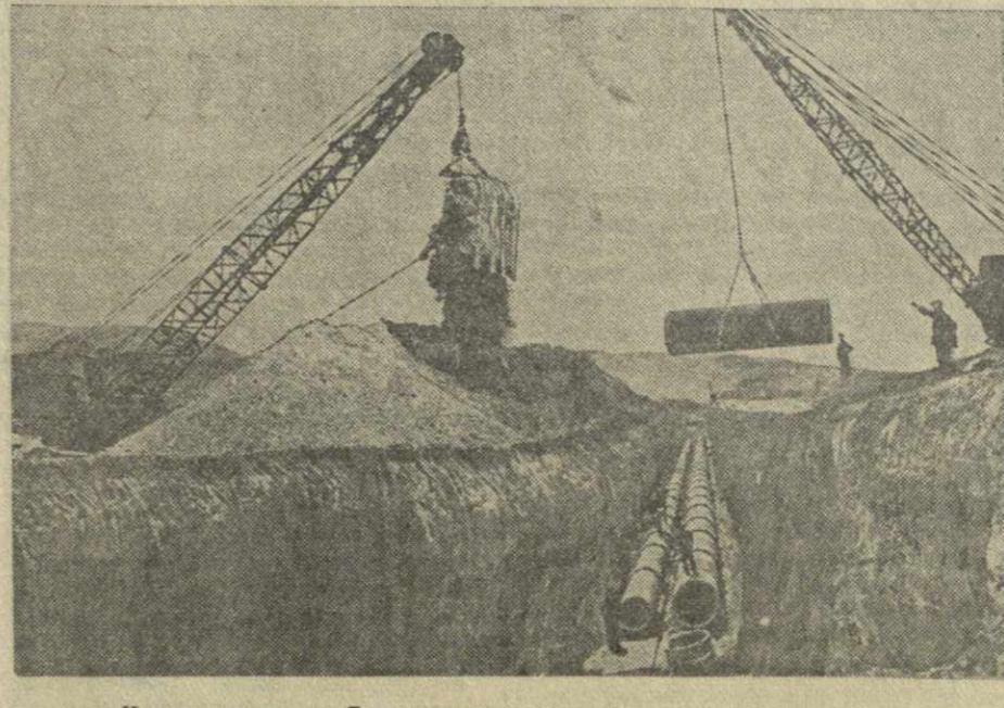
На строительстве Булачуурского водопровода. Фото М. Квирикашвили.
