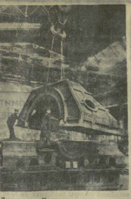
Ленинград. Коллектив завода имени Сталина работает над изготовлением паровой турбины высокого давления мощностью 50 тысяч киловатт. На снимке: сборка железной конструкции планшара турбины. На переднем плане — строитель Ф. И. Краснов (слева) и Ф. С. Семенов, выполняющие по две нормы за смену. Фото П. Федотова. (Фотокроника ТАСС).
