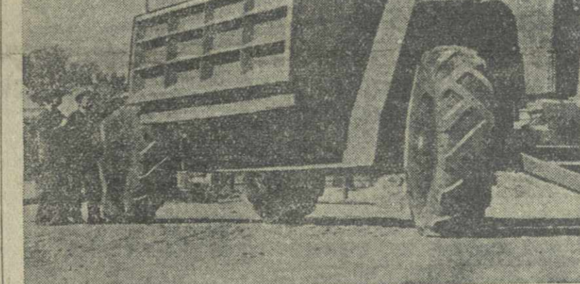
Харьков. Коллектив завода дорожных машин освоил выпуск нового большегрузного прицепа для земляных работ на крупных строительных площадках. Прицеп вмещает 15 кубических метров грунта и в течение 14 секунд разгружает его. Имея большую маневренность, прицеп может выгружать грунт на обе стороны. Новая машина заменяет около пяти автомашин грузоподъемностью до 5 тонн. Агрегат обслуживает один человек — водитель трактора.
