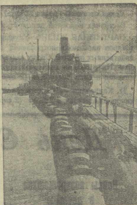
Литовская ССР. Коллектив Каунасского судоремонтного завода выпускает новый мощный землесосный снаряд. Испытания показали, что он заменит четыре пловучих многокошковых экскаватора и отводит пугулы на сотни метров. Новый агрегат слан рекордами для эксплуатации.
