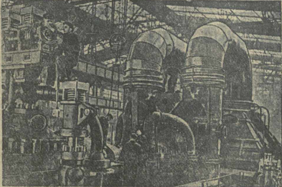
Коллективом Ленинградского металлического завода имени Сталина закончена сборка на стенде паровой турбины мощностью в 150 тысяч киловатт. На снимке: подготовка турбины к испытанию.
