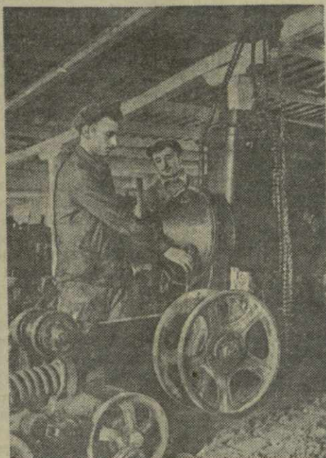
Механизаторы Цительской МТС ремонтируют тракторы передовым узловым методом. На снимках: 1. Кузнечный цех. В. Гоголашвили (слева) и К. Багров в пневматическом молоте. 2. Слесарно-сборочный цех. С. Арзуманян (слева) и Г. Мегребанов собирают задний мост трактора. 3. Токарный цех. Зав. мастерскими Н. Вербовский (в центре) проводит работу токаря В. Кунчина.
