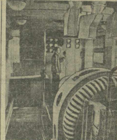
Челябинский автомеханический завод освоил выпуск вагонов-электростанций ВЭС-4. Эксплуатация смонтирована в четырехсотом вагоне, имеет двигатель мощностью 450 лошадиных сил и генератор мощностью 320 киловатт. Вагон-электростанция предназначена для работы на стройках.
