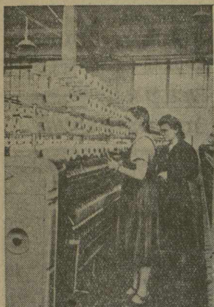
На ниточной фабрике Ташкентского текстильного комбината (Узбекская ССР) сейчас испытывается малогабаритная крутильная машина марки «К-66-1». На снимке: крутильщица А. Я. Шенцова за работой на малогабаритной крутильной машине «К-66-1». Справа — конструктор бюро Л. А. Сукакова.
