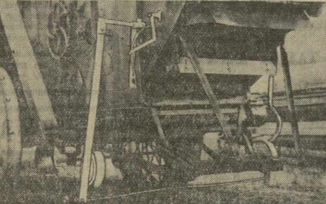
Балансирующее приспособление И. Чуаде, установленное на комбайне «Сталинец-6».
