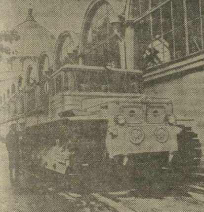
«ДЭТ-250» — таково название нового 250-сильного дизельэлектрического трактора, спроектированного и сооруженного на Челябинском тракторном заводе.
