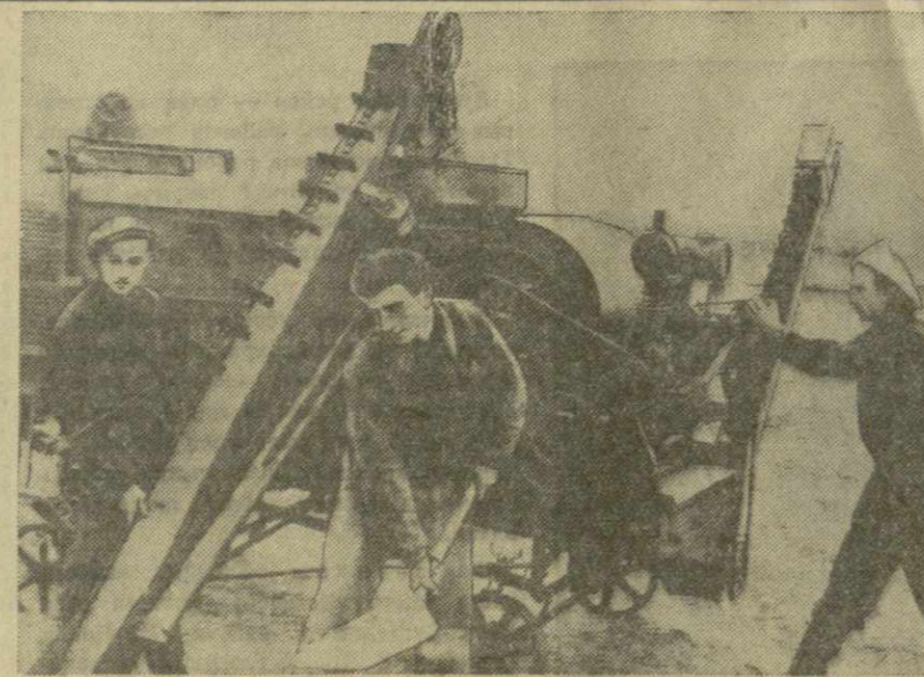
В кустанайской степи на уборке богатого урожая самоотверженно трудятся учащиеся Сухумского сельскохозяйственного техникума. На снимке (слева направо): Р. Званбая, О. Кочкаян, А. Чабрава, обслуживающие зерноочистительную машину «ОВ-10». Фото Х. Харлампиди.
