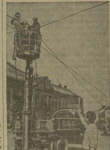
Вильнюс. В шестой пятилетке в Вильнюсе намечено провести больше работы по улучшению обслуживания трудящихся внутригородским транспортом. Сейчас ведется монтаж первой троллейбусной линии. На снимке: монтаж троллейбусной линии по улице Комюнина. Старший инженер треста «Мосэлектротранс» Михаил Панасенко (справа) дает указания монтажникам Николаю Михалевичу и Григорию Толпалову. Фото Л. Мейнерта. Фотохроника ТАСС.
