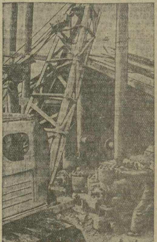
Сахалинская область. Монтажные работы на строительстве буровых вышек нефтяных промыслов Сахалина полностью механизированы. Здесь применяются бульдозеры, тракторные подъемные краны, электроподъемные лебедки.
