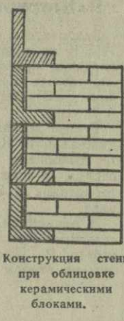
Конструкция стены при облицовке керамическими блоками
