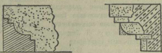
БЛОЧНЫЙ КАРНИЗ КАРНИЗ ИЗ ОТДЕЛЬНЫХ ЭЛЕМЕНТОВ СЕЧЕНИЕ КАМНЯ СЕЧЕНИЕ КАМНЯ, УДАЛЯЕМОГО ПРИ ОБРАБОТКЕ ЖЕЛЕЗОБЕТОННАЯ ОСНОВА
