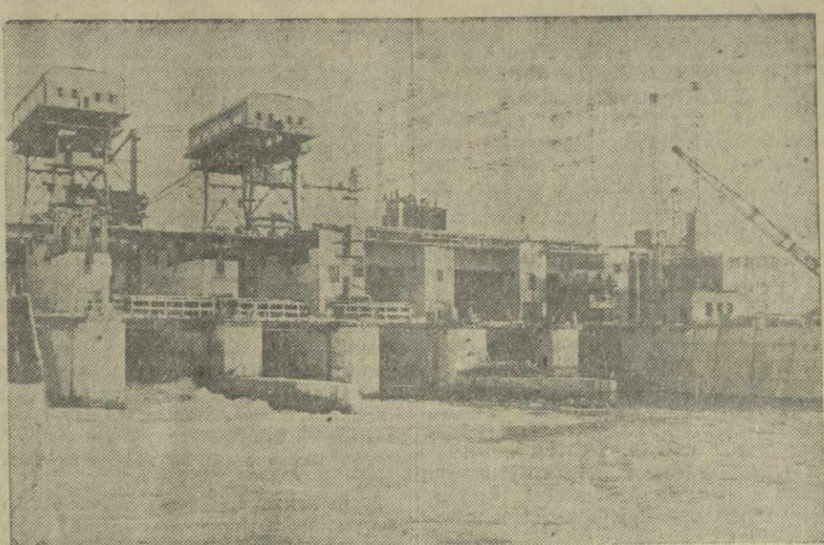
Таджикская ССР. На снимке: вид гидроузла Кайрак-Кумской ГЭС с нижнего бьефа. Фото А. Полякова. Фотохроника ТАСС.
