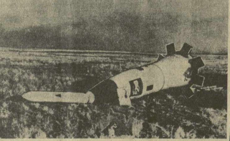
Советские ученые провели в последнее время ценнейшее исследование верхних слоев атмосферы и явлений, происходящих в космическом пространстве.
