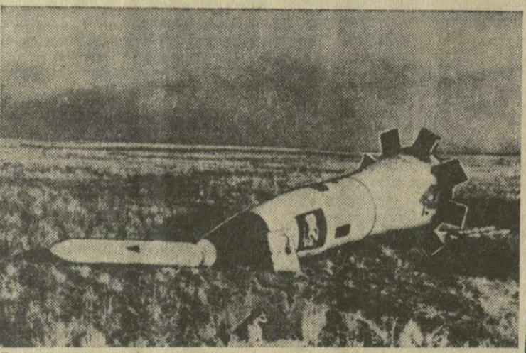
Советские ученые провели в последнее время ценнейшее исследование верхних слоев атмосферы и явлений, происходящих в космическом пространстве.
