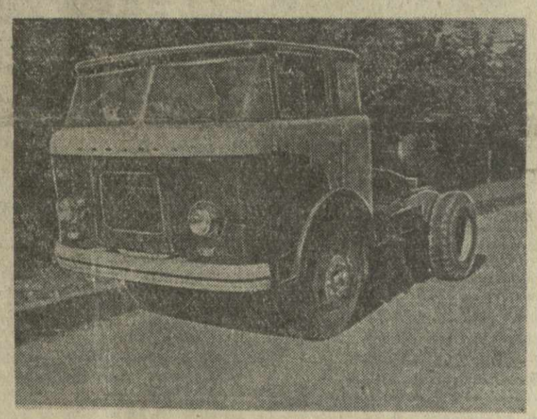
Конструкторы Кутаисского автозавода имени Г. К. Орджоникидзе совместно с коллективом экспериментального цеха создали опытный образец тягача нового типа «КА3-606», серийный выпуск которого предусмотрен в 1960 году. Новый тягач располагает двигателем мощностью в 110 лошадиных сил, он может перевозить 8 тонн грузов. В кабине машины два места и одно спальное место для запасного водителя.
