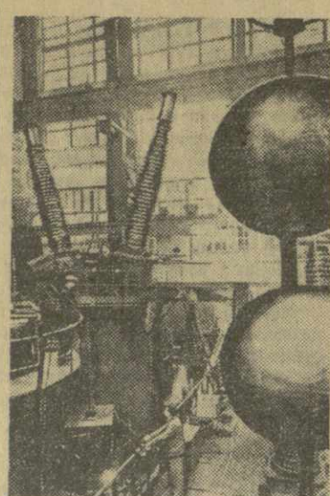
На свердловском заводе «Уралэлектротраппарат» закончена сборка и проводится испытание нового мощного масляного выключателя на 500.000 вольт. Этот выключатель предназначен для линии электропередачи Волжская ГЭС имени В. И. Ленина—Урал.
