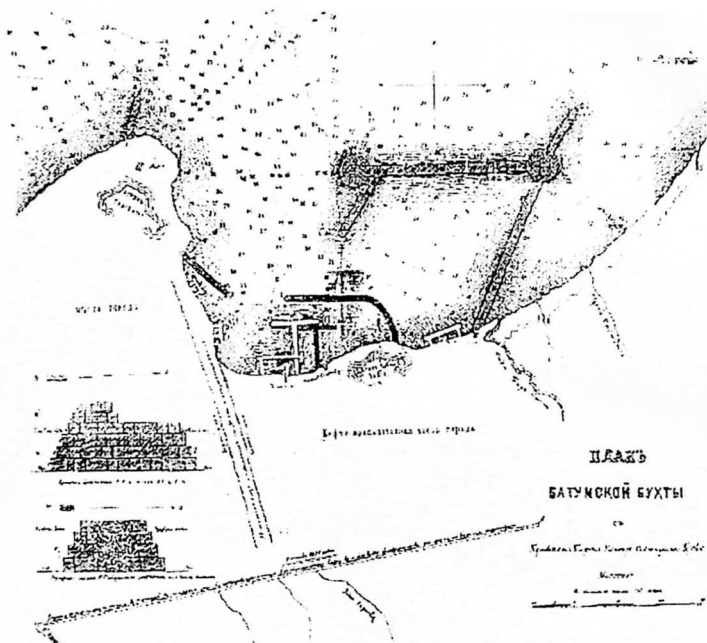
ბათუმის პორტის პროექტი (ავტორი ა. გრევე), 1882 წ.
