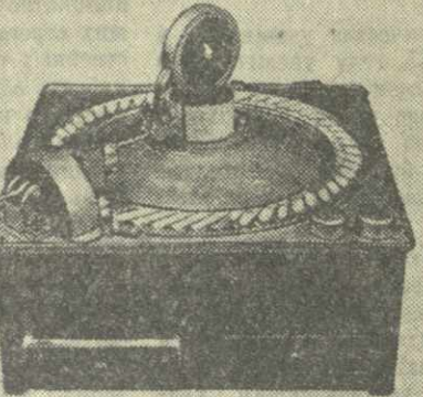
На верхнем снимке — регистрирующая часть автомата: диаграмма сортировки и циферблат, на котором отсчитывается величина средней сортировки всей испытываемой партии коконов.
