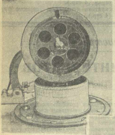
На нижнем снимке вы видите общий вид прибора-автомата КБ-1. Автомат включает диск, вращающийся, и коконы, разложенные в ячейки, проба испытание под площадкой сжатия, падают в левый ящик.
