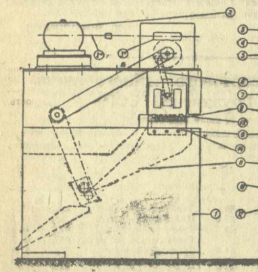
Схема универсального станка для изготовления двустороннего ножовочного полотна.
