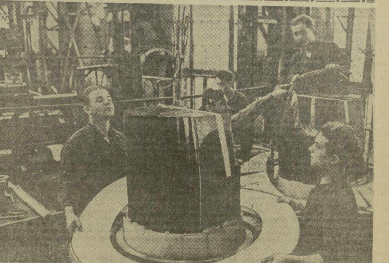
Московские трансформаторостроители заканчивают изготовление крупного трансформатора для одной из электростанций Грузии. Мощность этой машины 23 тысячи киловатт-ампер напряжением 220 тысяч вольт. На снимке: на сборке трансформатора. На переднем плане — сборщики А. Орехов (слева) и В. Завражков, выполняющие ежедневно по два сменных задания. Фото В. Кунова, (Фотохроника ТАСС).
