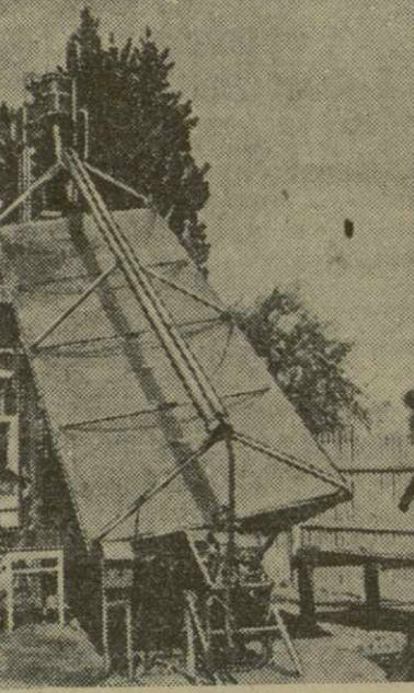
Устройство солнечной параболо-цилиндрической котельной, установленной в Ташкенте, на экспериментальной базе Энергетического института Академии наук СССР.
