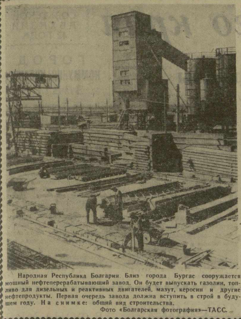
Народная Республика Болгария. Вокруг города Бургас сооружается мощный нефтеперерабатывающий завод. Он будет выпускать газولين, топливо для дизельных и реактивных двигателей, мазут, керосин и другие нефтепродукты. Первая очередь завода должна вступить в строй в будущем году. На снимке: общий вид строительства. Фото «Болгарская фотография»-ТАСС.
