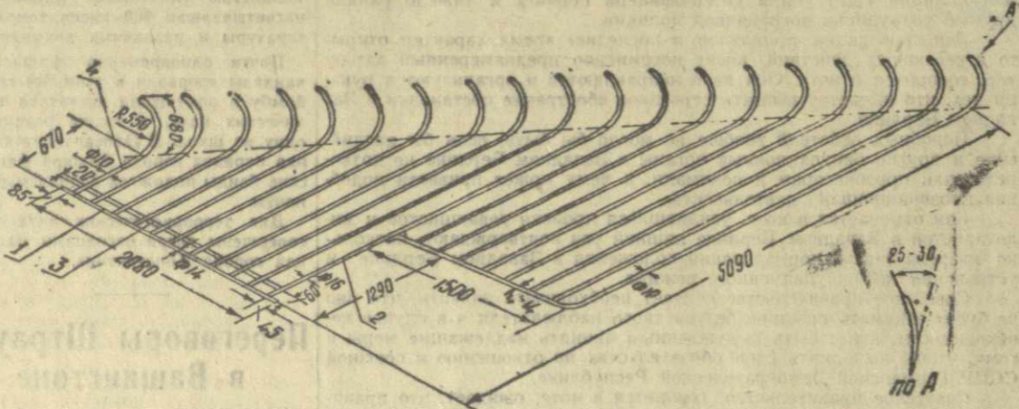
Рис. 1. Уширенный валкообразователь.
