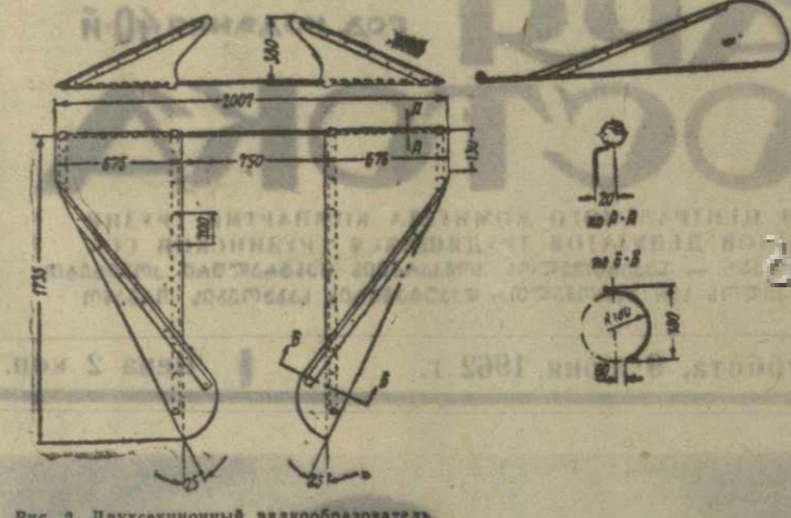
Рис. 2. Двухсекционный валкообразователь.
